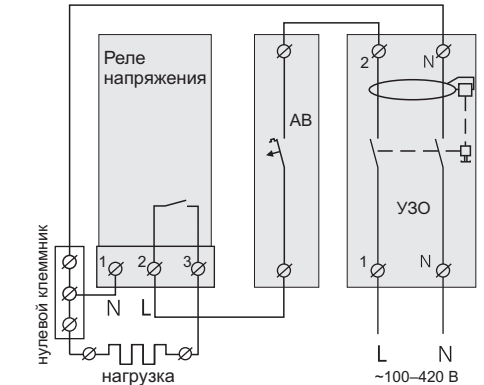
Схема 2. Подключение автоматического выключателя и УЗО
