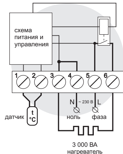
Схема 1. Схема подключения и упрощенная внутренняя схема
